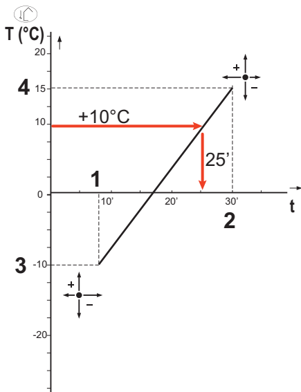
Fig.96 Courbe de temporisation du démarrage de l'appoint
