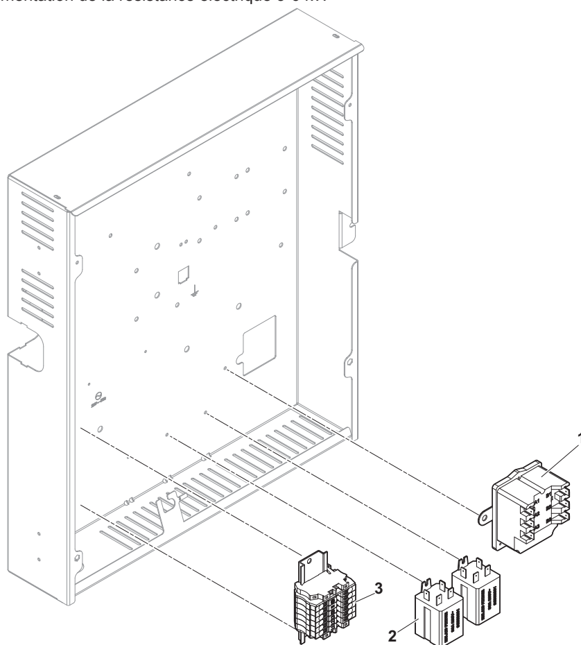
Fig.183 Alimentation de la résistance électrique 3-6 kW
