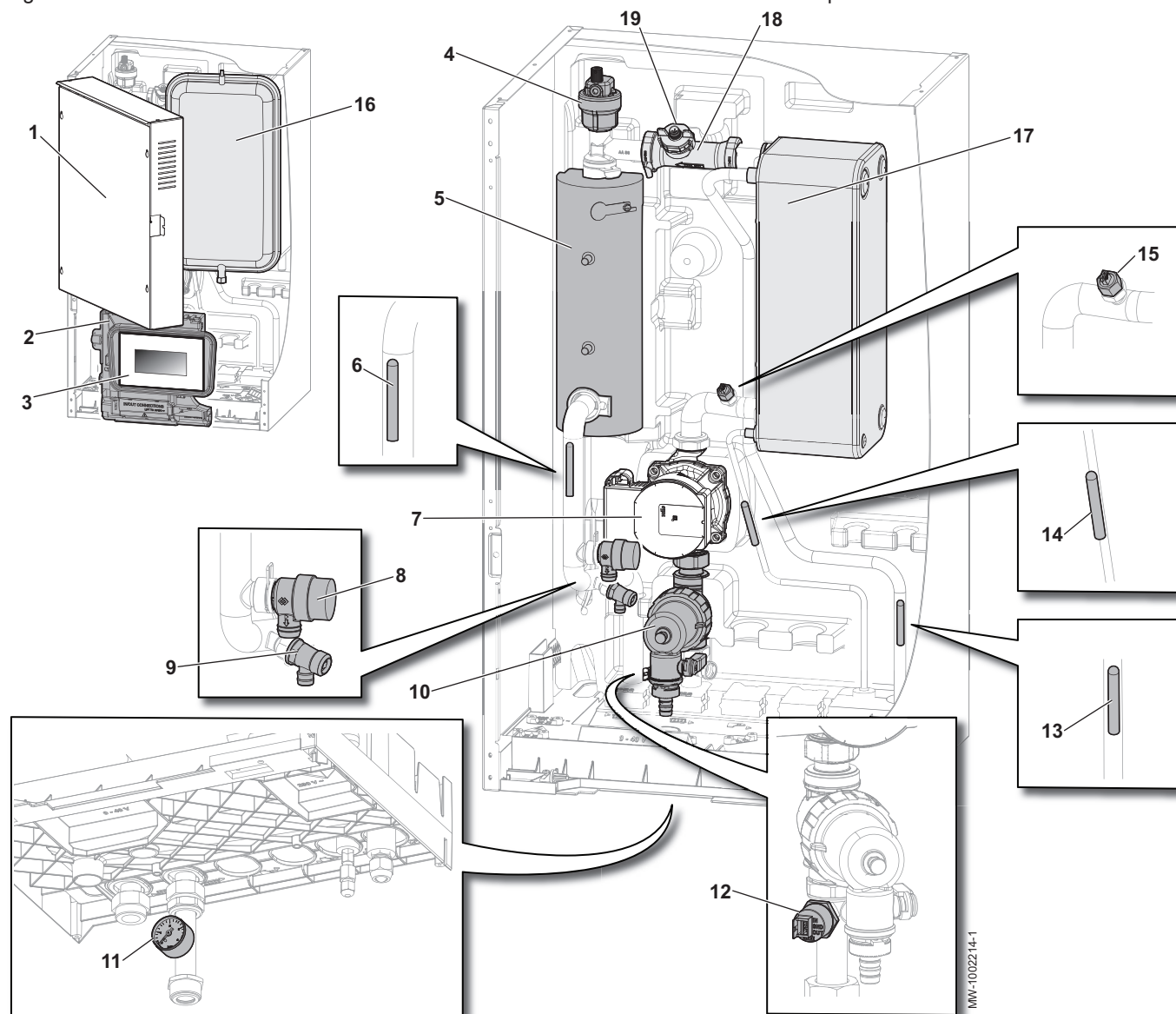
Fig.16 Module intérieur Mod. Int. ERIA S PLUS 12-16/EM R32 avec résistance électrique
