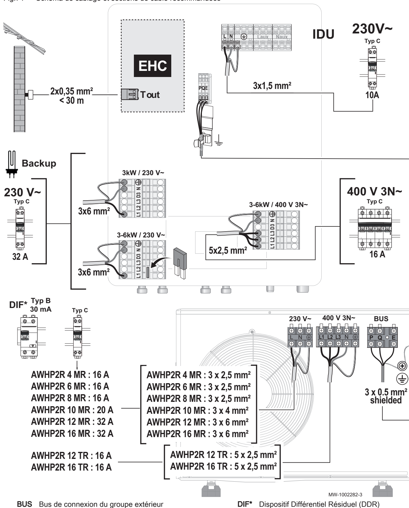
Fig.74 Schéma de câblage et sections de câble recommandées
