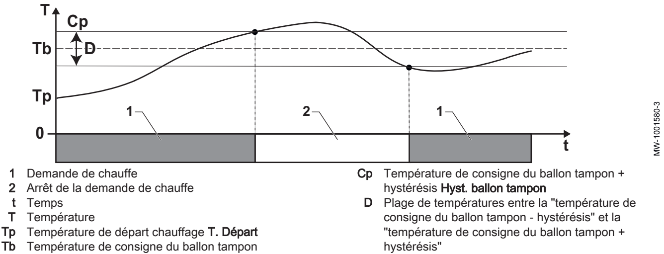
Fig.98 Logique de basculement de la demande de chauffe du ballon tampon
