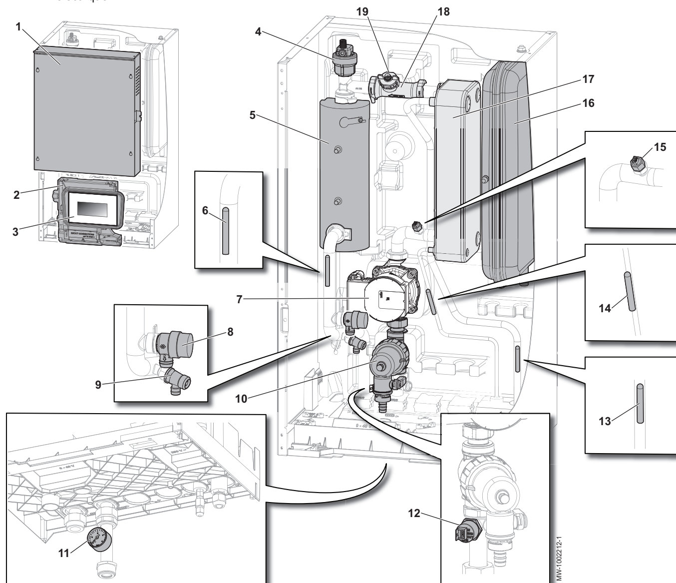
Fig.15 Module intérieur Mod. Int. ERIA S PLUS 4-6/EM R32 et Mod. Int. ERIA S PLUS 8-10/EM R32 avec résistance électrique
