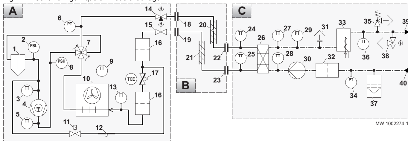
Fig.12 Schéma frigorifique en mode chauffage
