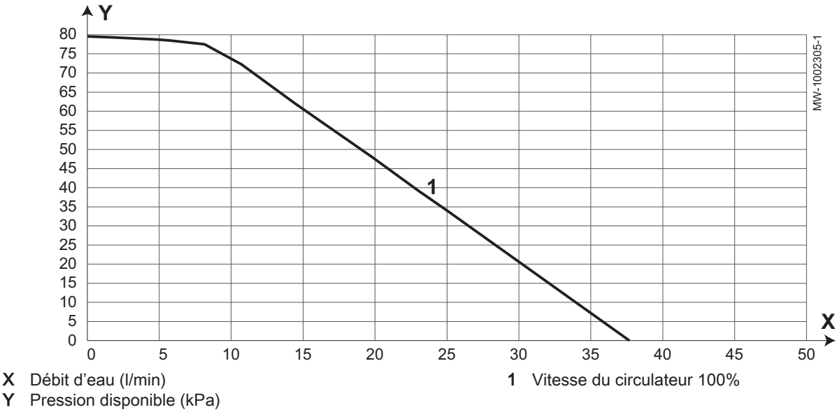
Fig.7 Pressions disponibles 4-10 kW
