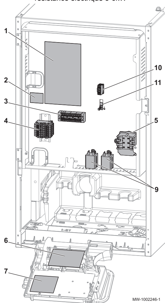
Fig.17 Emplacement des cartes électroniques - version avec résistance électrique 3-6kW
