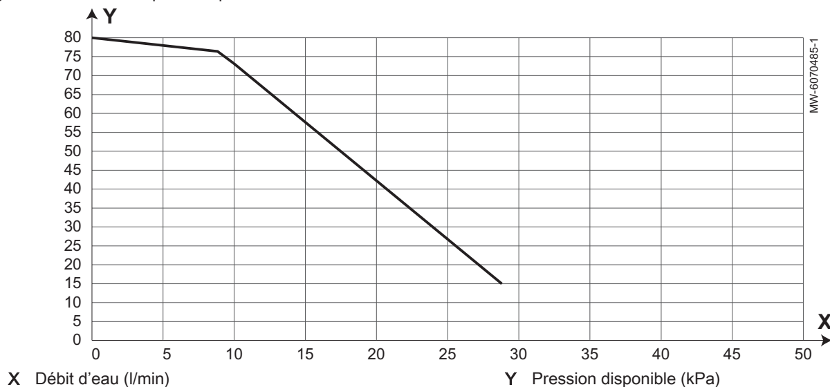
Fig.5 Pressions disponibles pour iMPI/E 4-8 iR32 + AWHPR 4 -8MR
