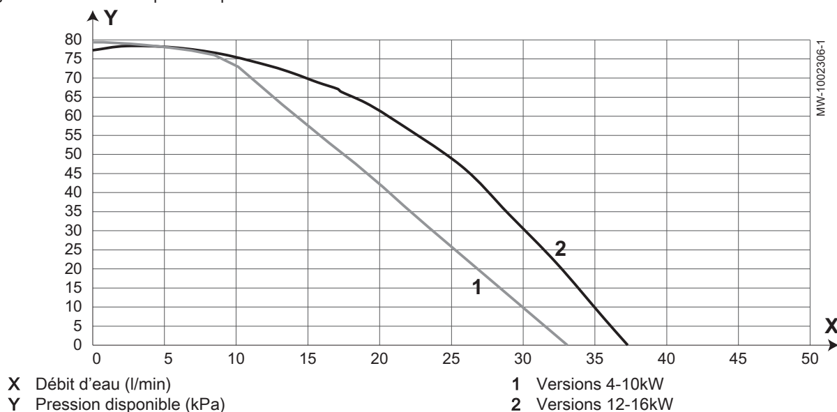
Fig.6 Pressions disponibles pour Mod. Int. ERIA S PLUS + AWHP2R et iMPI/E iR32 M + AWHP2R
