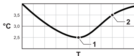
Fig.49 Comportement de la protection antigel
