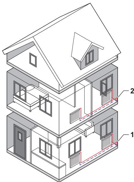
Fig.6 Deux circuits de chauffage
